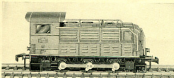
635 - Loco diesel de manœuvre C 61006. Longueur 130 mm.
