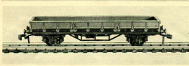
718 - Wagon à ridelles basses - Longueur 128 mm
