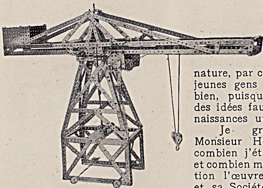
Grue à Roulement Radial
