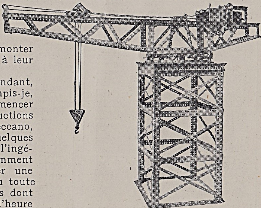
Grue à Flèche Horizontale
