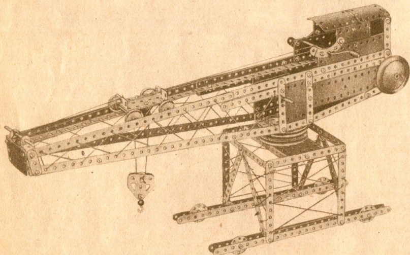
Grue géante à flèche horizontale
