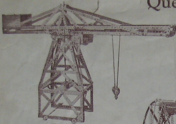
Grue à Roulement Radial
