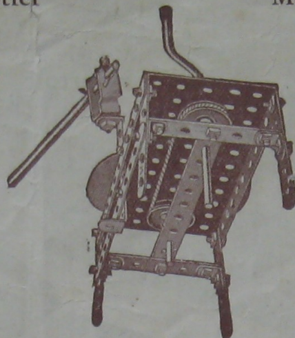
Tour de Potier (vue par-dessous)
