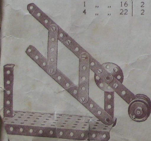
Modèle No. 25— Barrière de Passage à Niveau
