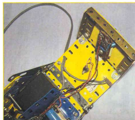
Diverses vues du butoir montrant l'implantation de l'électronique et de sa commande
