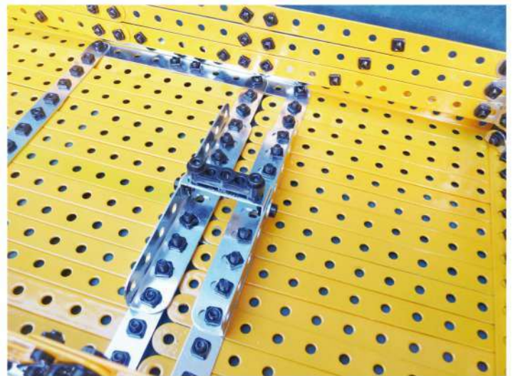
Fig. 24 Le palier inférieur
