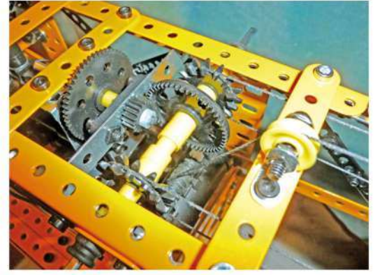
Fig. 15 Le treuil et la commande du chariot
