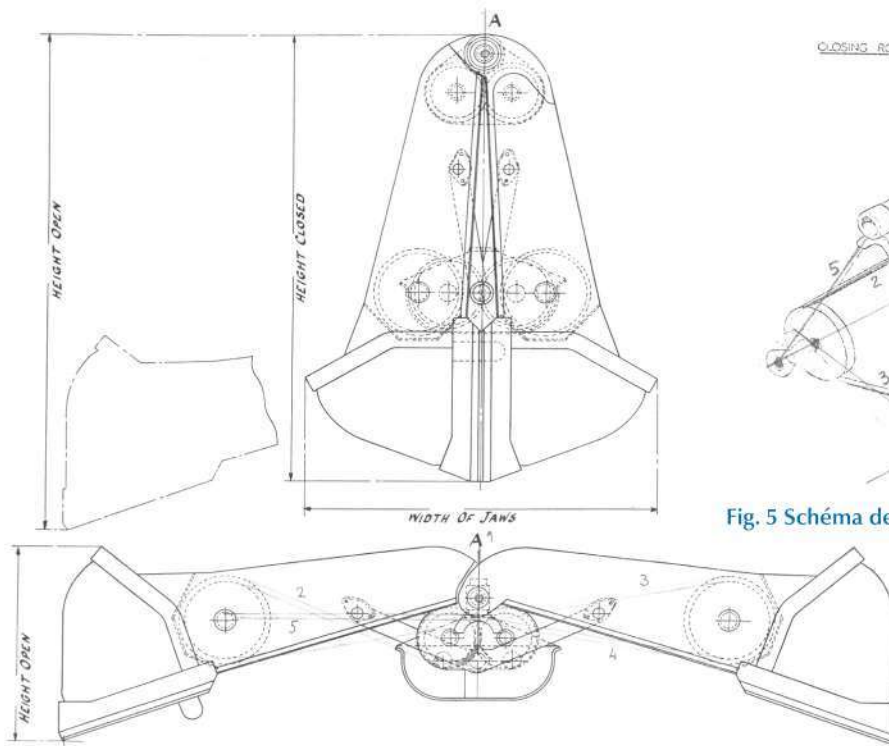
Fig. 4 Schéma de principe de la benne Trojan, câbles de suspension
