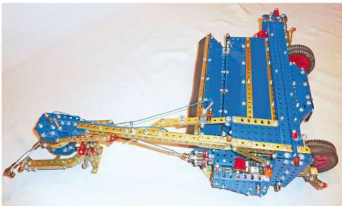
Fig. 17 Faucheuse vue de gauche
