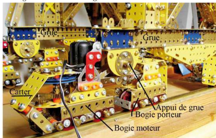
Fig. 5 Chariot mixte à simple bogie moteur et bogie porteur
