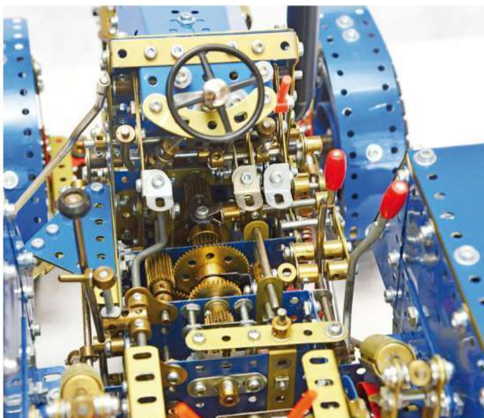
Fig. 8 Poste de pilotage
