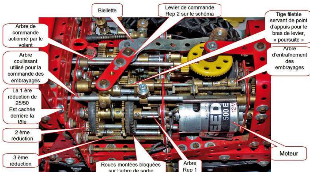
Fig. 5 Direction assistée sur le Latil
