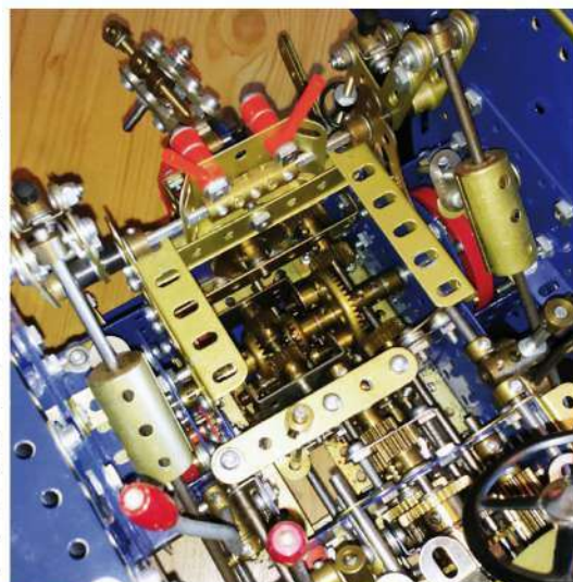
Fig. 10 Entraînement de la prise de force
