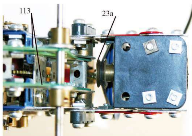
Fig. 12 Vue de la poulie 23a
