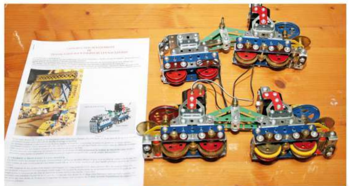
Fig. 10 Essieux motorisés d'Yves Boissel
