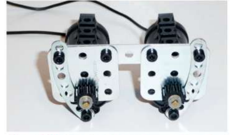
Fig. 28 Fixation des 2 autres moteurs sur des plaques 3x3 trous
