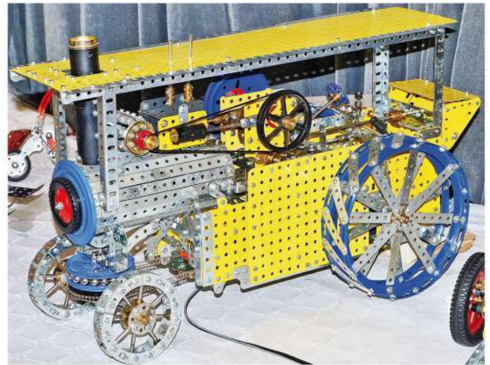
Fig. 11 Un ancien tracteur à vapeur, animé, de Jean-René
