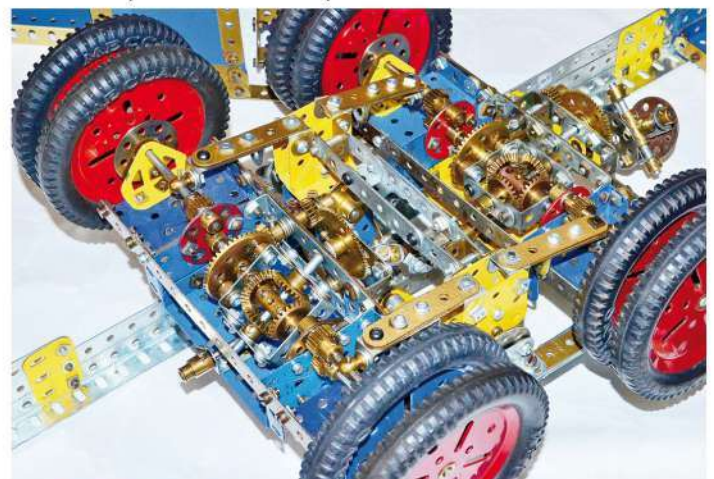
Fig.13 Pont arrière jumelé de camion de Bernard Journaux
