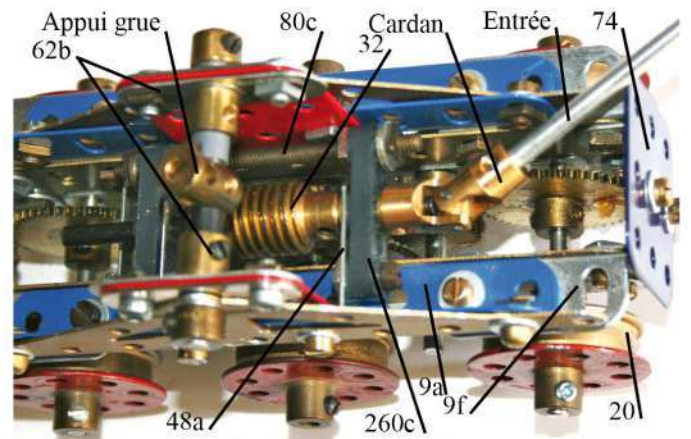
Fig. 2 Chariot vu de dessus
