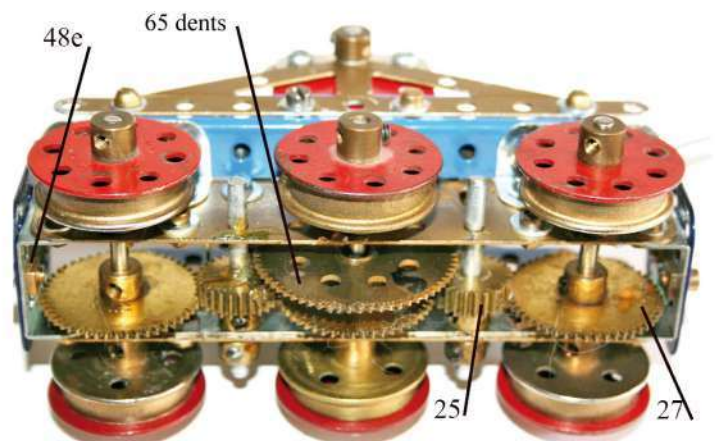
Fig. 4 Chariot vu de dessous
