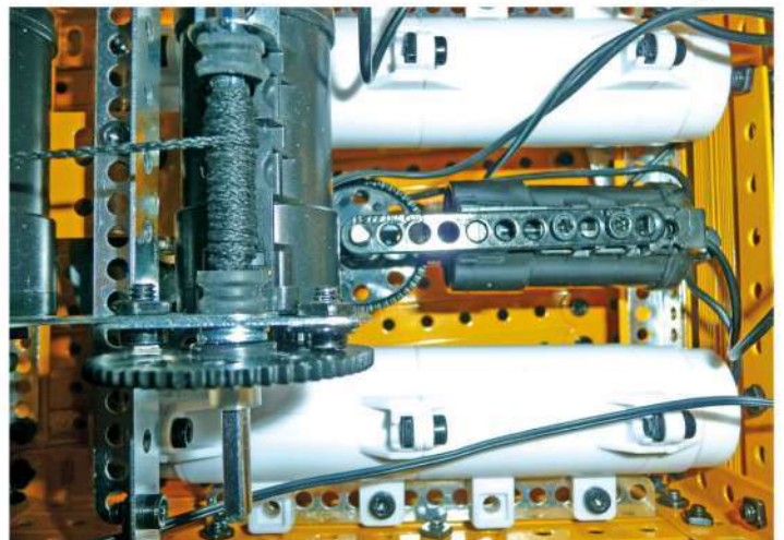
Fig. 31 L'intérieur de la cabine avec les boîtiers de piles et les moteurs
