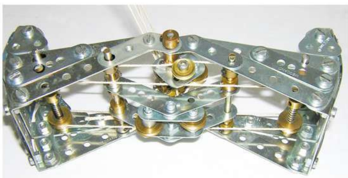
Fig. 6 Benne ouverte
