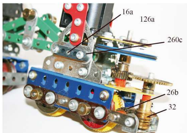
Fig. 10 Détail de la transmission
