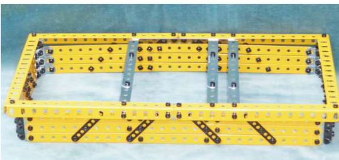
Fig. 22 Construction de la barge, la coque
