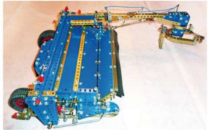
Fig. 14 Faucheuse vue de droite
