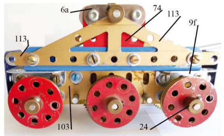
Fig. 3 Chariot vu de face
