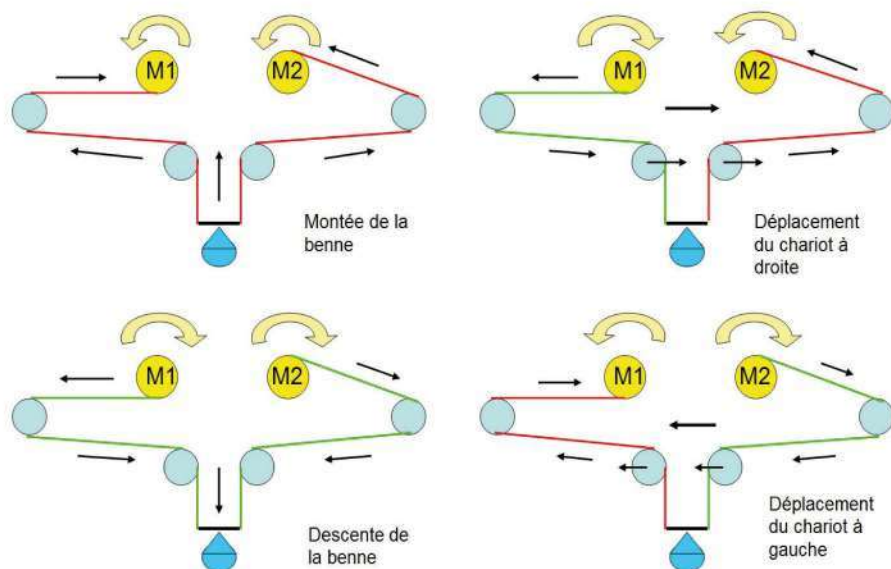
Fig. 1 Schéma de principe du système Caillard
