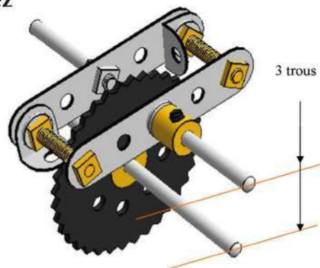
Fig. 2 Espacement de 3 trous entre les deux axes
