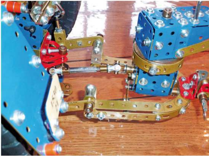
Fig. 13 Attache de la faucheuse sur le tracteur
