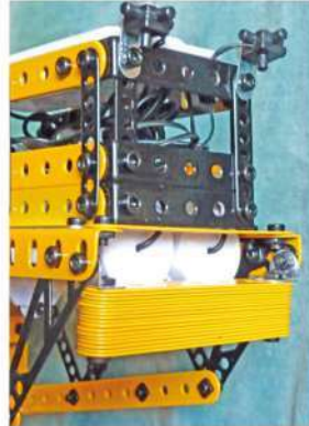
Fig. 7 Arrière de la cabine et contrepois
