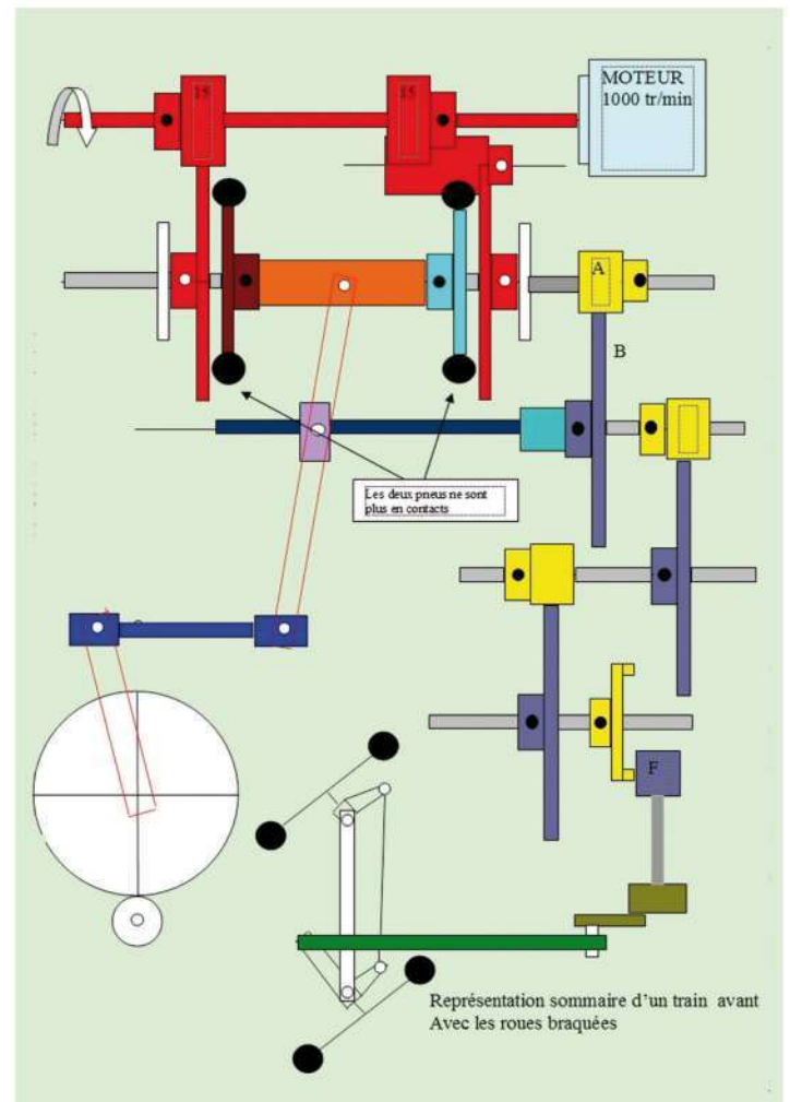
Fig. 3 Moteur en marche Plus d'action sur le volant Les deux pneus ne sont plus en contact
