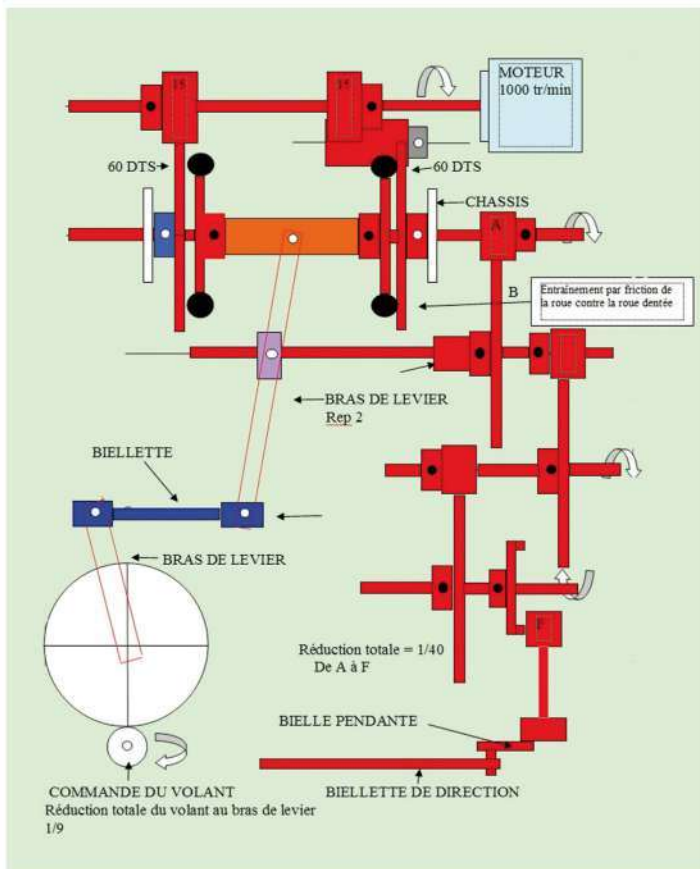
Fig. 2 Moteur en marche et rotation du volant en rouge les parties entraînées
