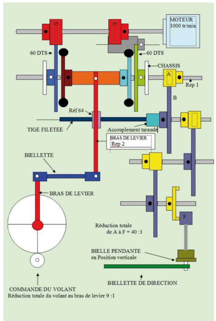
Fig. 1 Synoptique de l'ensemble
