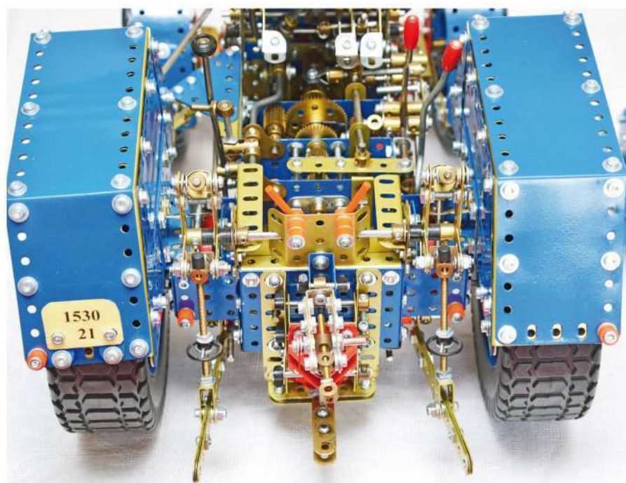
Fig. 9 Vue arrière du tracteur
