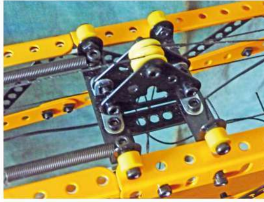
Fig. 14 Le chariot
