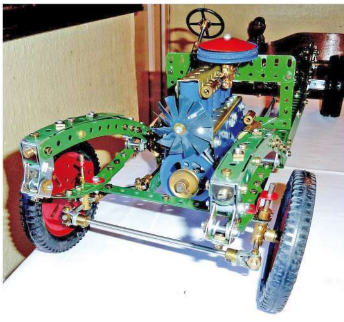
Châssis automobile par Christian Alain
