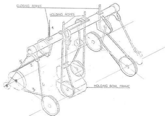
Fig. 5 Schéma de principe de la benne Trojan, câbles de fermeture
