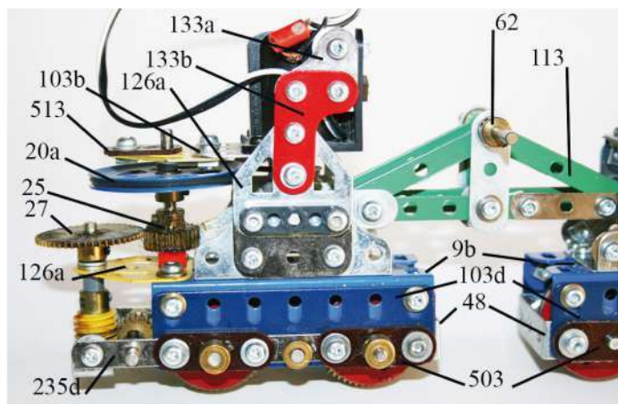
Fig. 7 Suite cinématique
