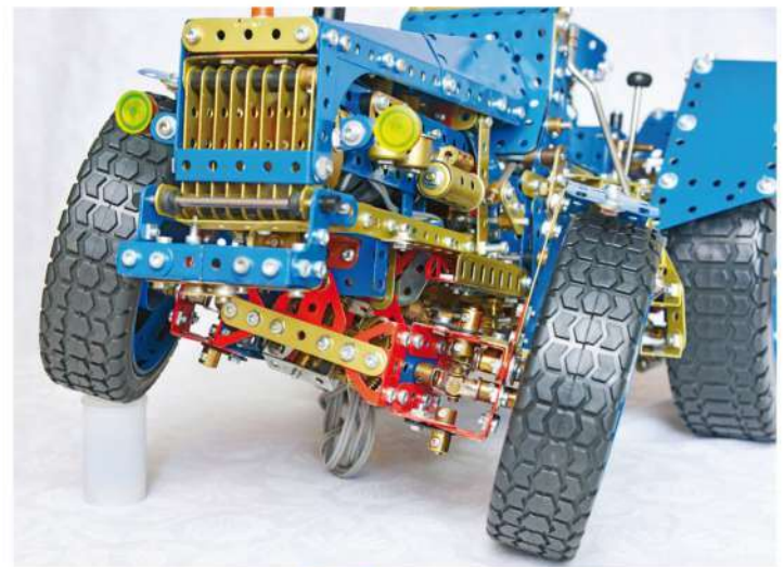
Fig. 4 Pont avant
