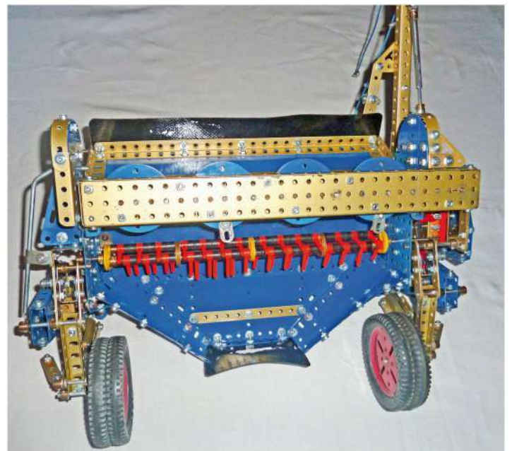
Fig. 16 Conditionneur à fléaux et lamier
