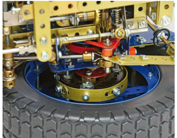
Fig. 7 Frein à expansion intérieure
