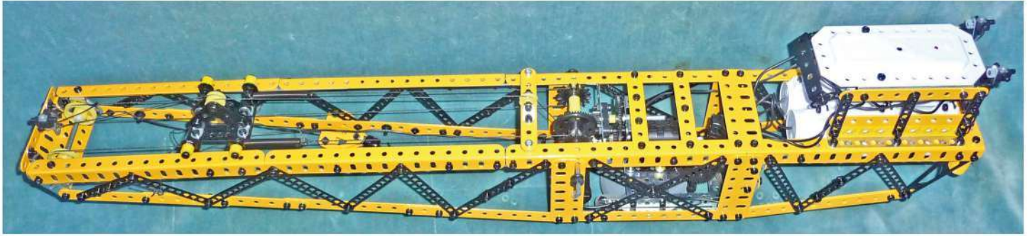
Fig. 5 La flèche horizontale et la cabine
