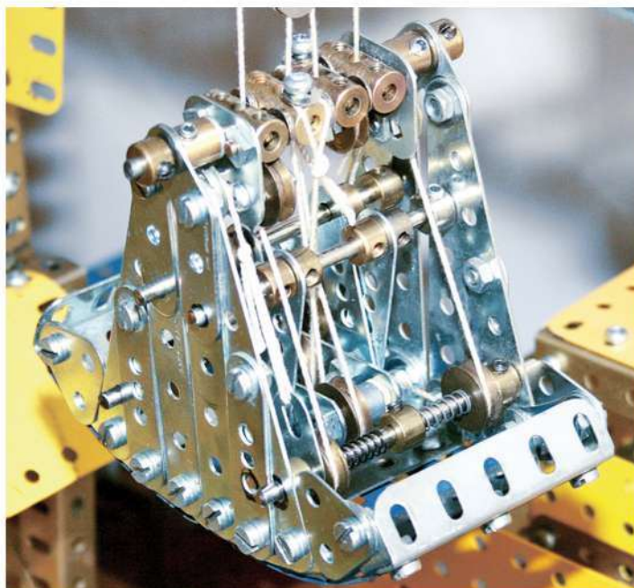
Fig. 7 Benne fermée
