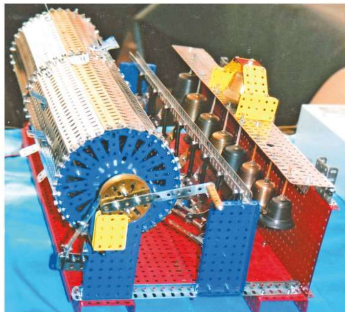
Fig. 2 Cylindre musical
