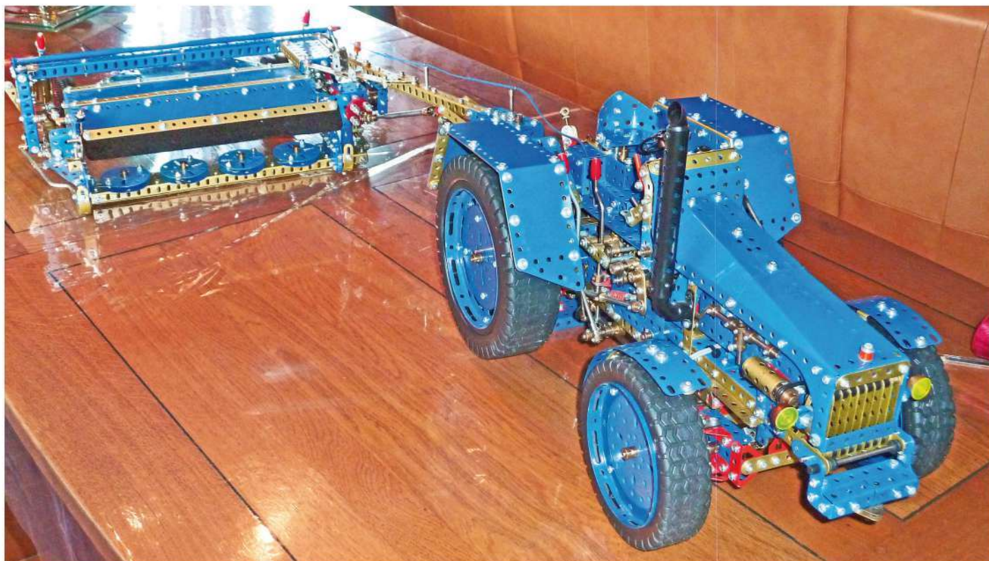
Fig. 12 Tracteur tractant la faucheuse à disques
