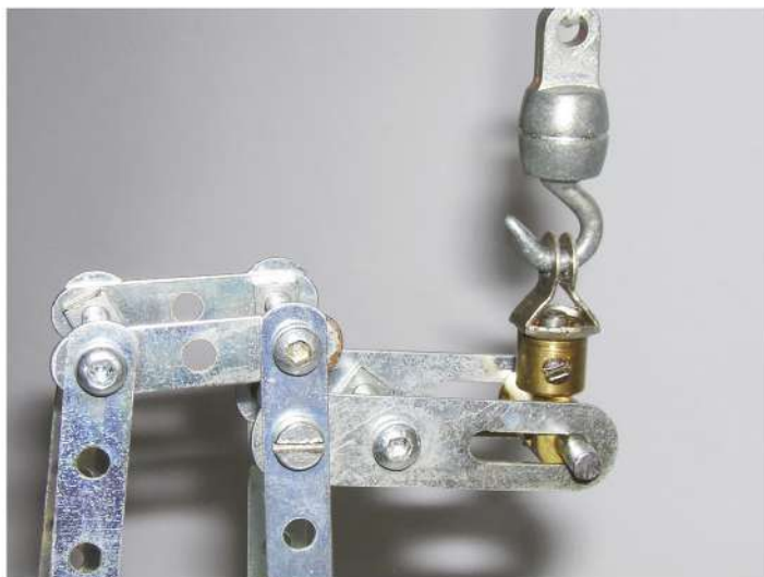
Fig. 3 Pièce de soulèvement
