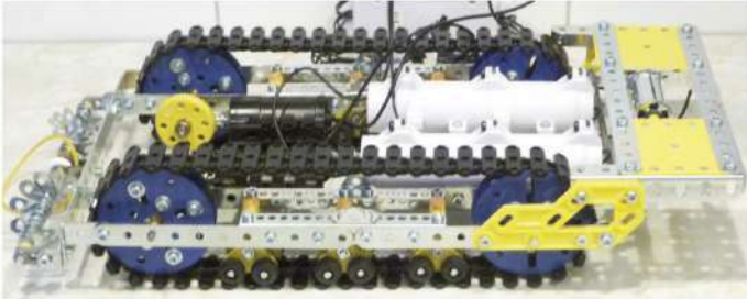
Fig. 10 Le châssis
