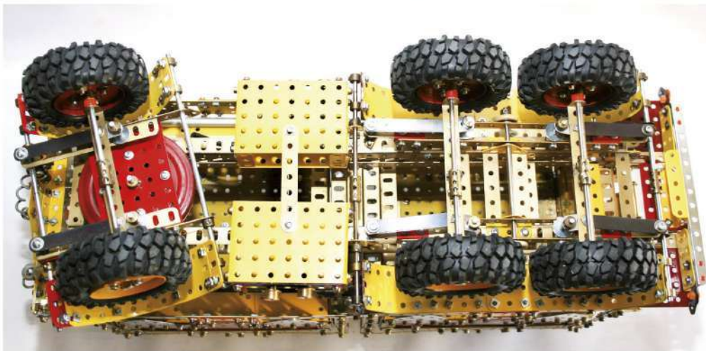
Fig. 12 Vue de dessous de la remorque
