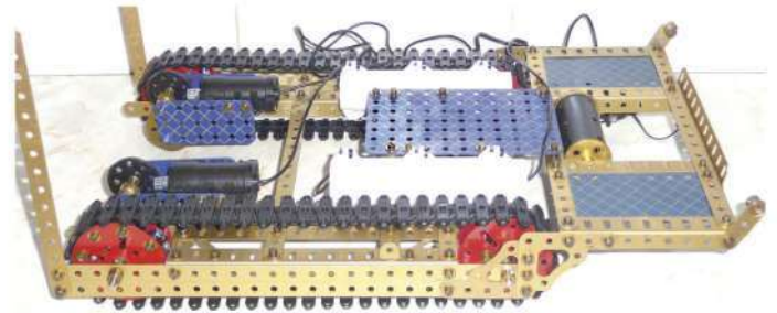
Fig. 2 Le châssis avec les nouvelles chenilles
