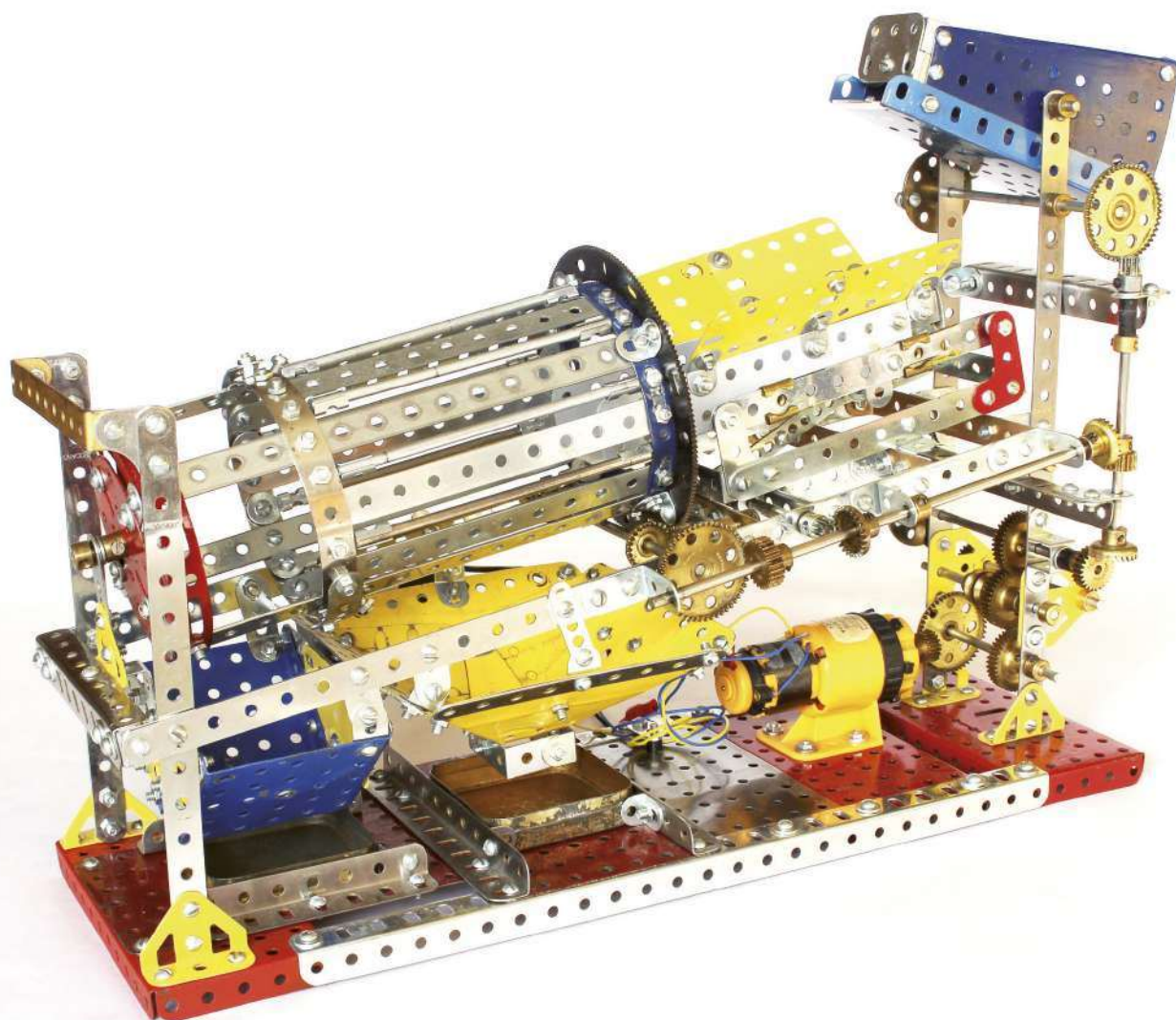
Fig. 1 Trieuse
