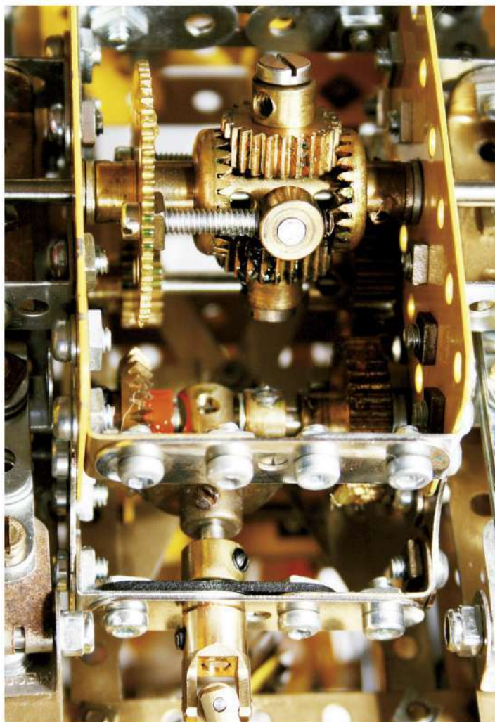
Fig. 6 Différentiel du tracteur
