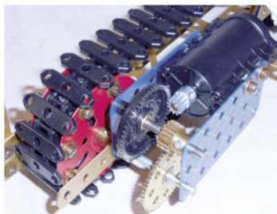
Fig. 4 Le moteur entraînant la chenille
