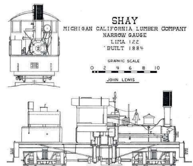
Fig. 2 Schéma Shay
