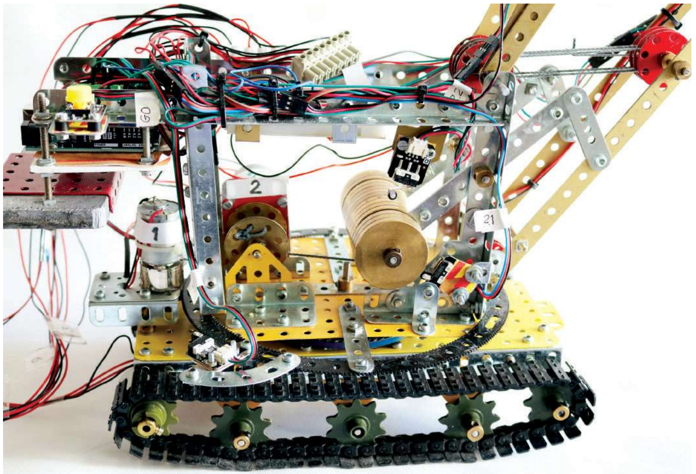
Fig. 5 Moteurs 1 et 2 avec son treuil devant et le mouflage en haut à droite
