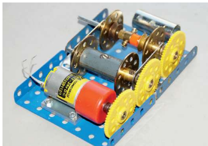
Fig. 8 Un aperçu de la conception du treuil du chariot bleu et de son moteur.
