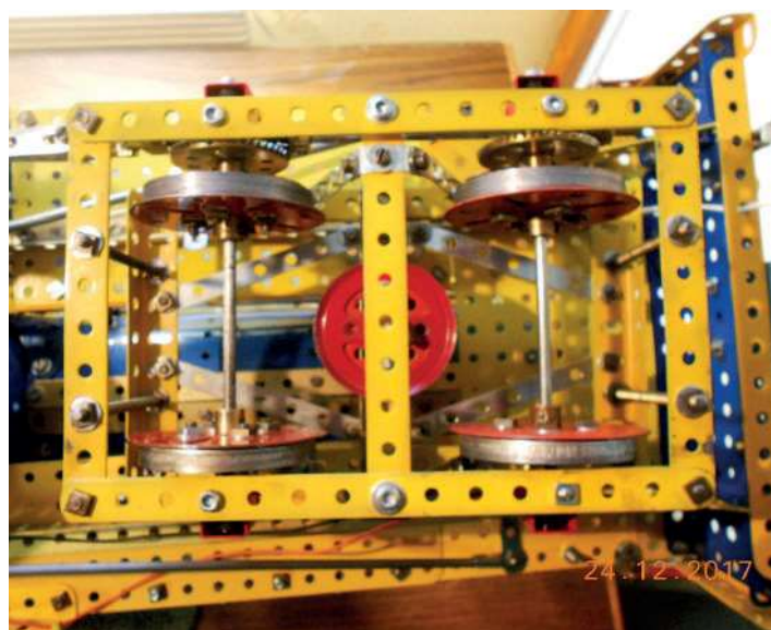
Fig. 10 Bogie vue de dessous
