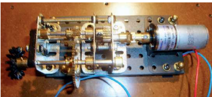
Fig. 14 Moteur et réducteur
