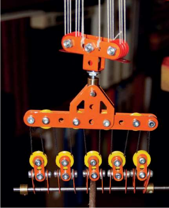
Fig.9 Un des palonniers associé à ses deux moufles à 16 brins. Moufle qui permet de lever en douceur 2kg sans effort apparent
