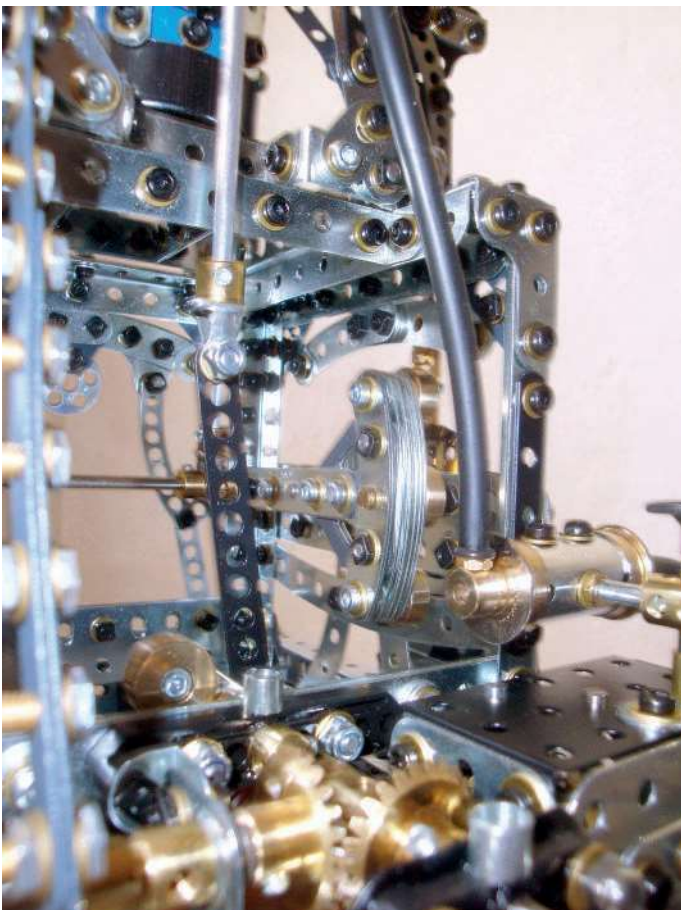
Fig. 8 Au centre, partie du vilebrequin et son contrepoids. Au premier plan transmission conique de la distribution
