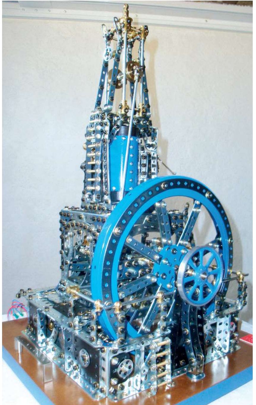
Fig. 10 Vue d'ensemble du volant d'inertie
