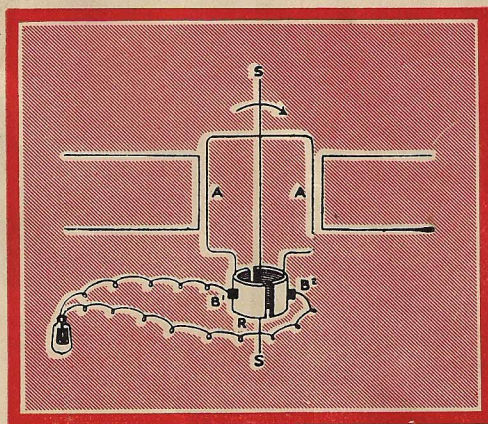
Fig. 36. Diagramme de Dynamo produisant un courant continu.
