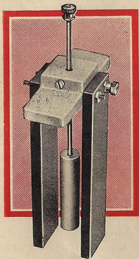
Fig. 6. Montage de la Pile au Bichromate Elektron avec la Tige de Zinc et les Plaques de Charbon en position.
