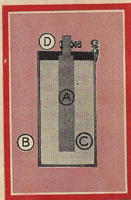
Fig. 4. Coupe d'une pile sèche.
