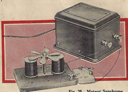
Fig. 39. Moteur Synchrone.
