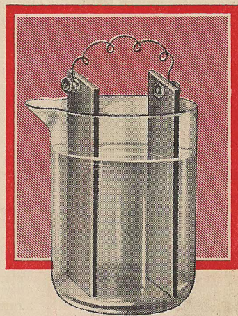
Fig. 2. Élément voltaïque.
