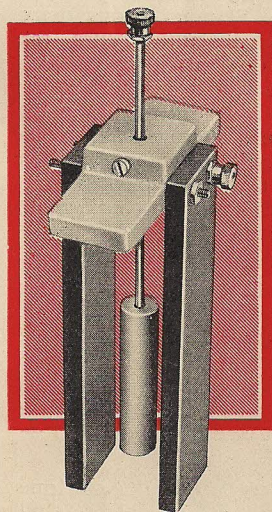
Fig. 6. Montage de la Pile au Bichromate de Potassium avec la Tige de Zinc et les Plaques de Charbon en position.
