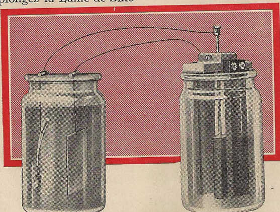
Fig. 41. Cuivrage d'une cuiller à l'aide d'un courant produit par la Pile au Bichromate Elektron.
