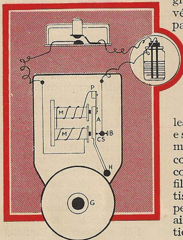
Fig. 20. Diagramme montrant le fonctionnement d'une sonnette électrique.
