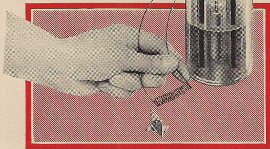
Fig. 16. Essai des propriétés magnétiques d'un solénoïde.
