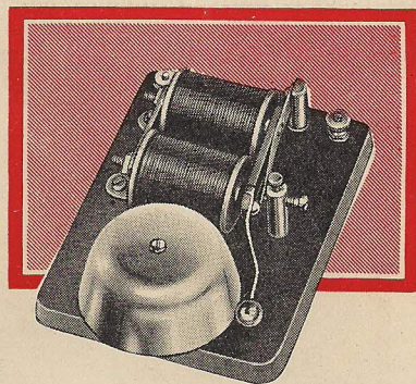
Fig. 23. Sonnerie électrique Elektron.
